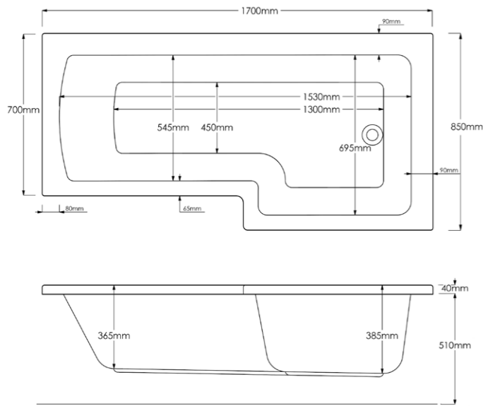
L-Shape
